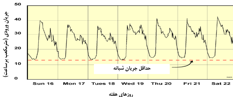
شکل ۱-۷- حداقل جریان شبانه در یک شبکه
